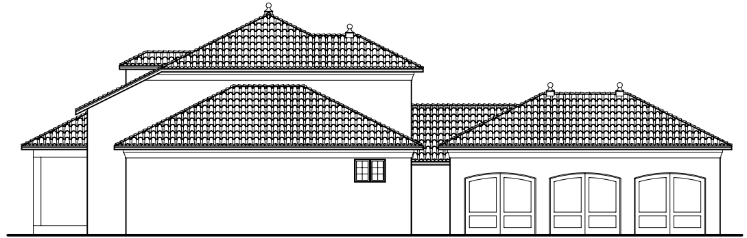
E2 LEFT ELEVATION
