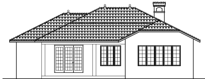
E3 REAR ELEVATION
