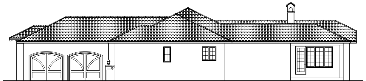
E4 RIGHT ELEVATION
