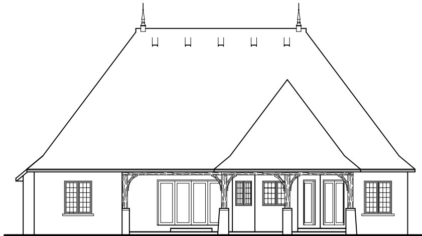
E3 REAR ELEVATION
