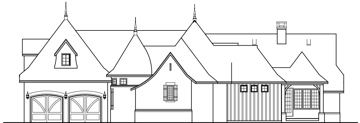
E4 RIGHT ELEVATION
