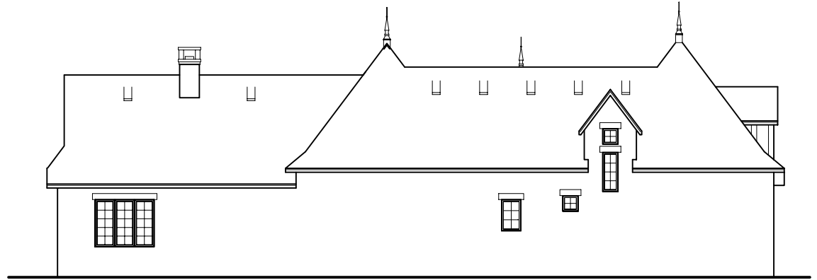
E2 LEFT ELEVATION
