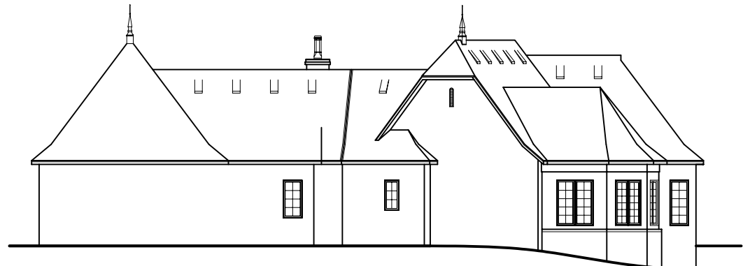
E4 RIGHT ELEVATION
