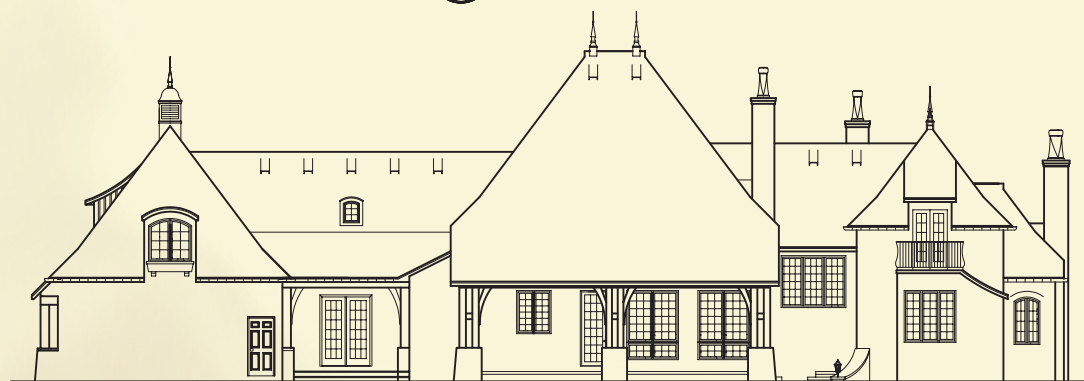
E3 REAR ELEVATION
