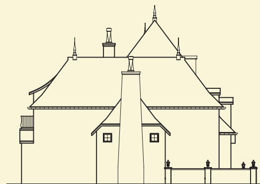
E2 LEFT ELEVATION
