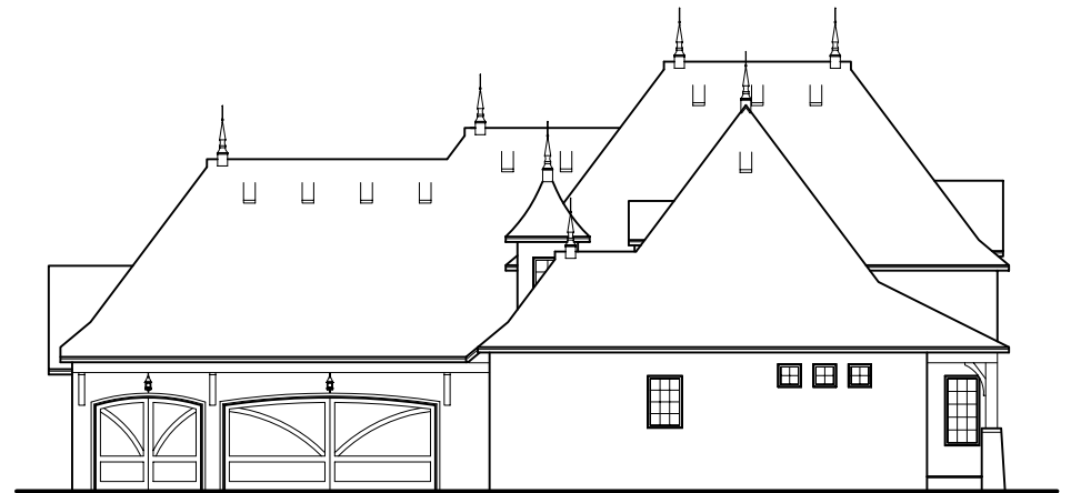
E4 RIGHT ELEVATION
