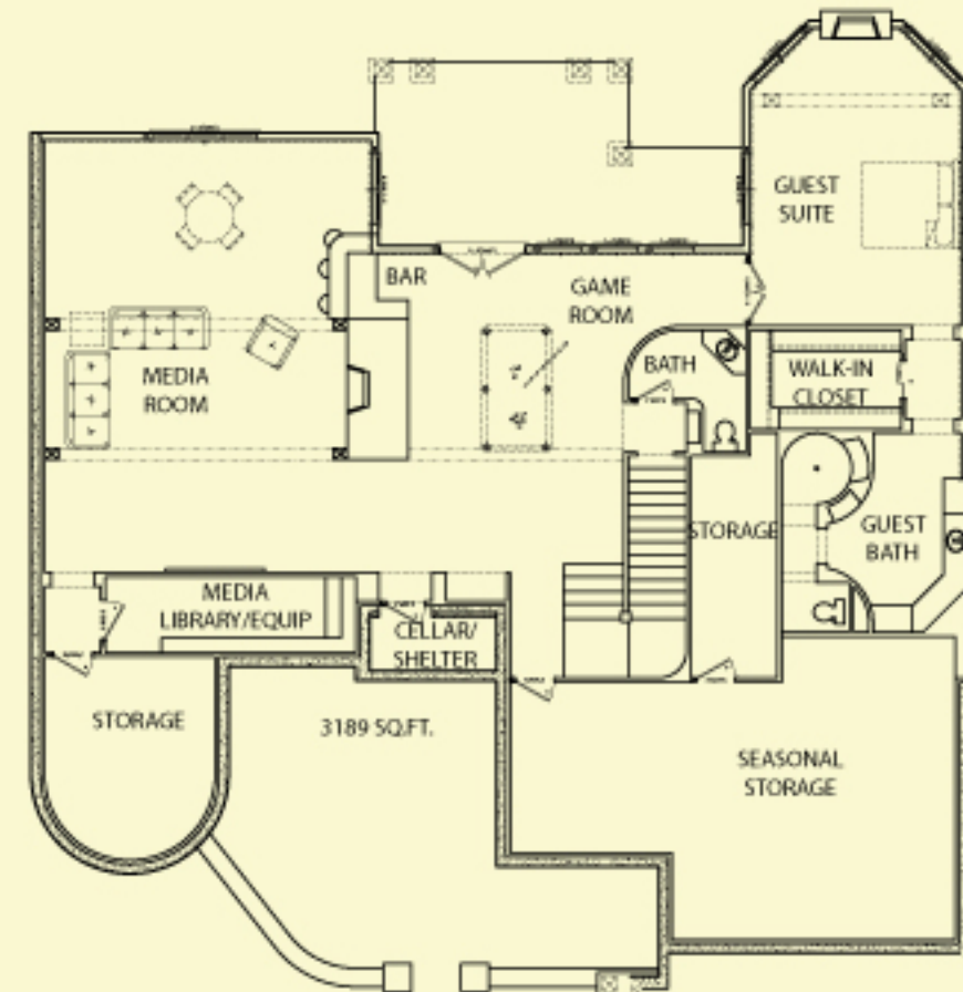
A5 BASEMENT
